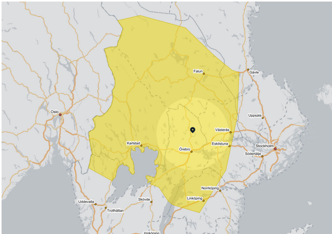
Grafik: SMHI
